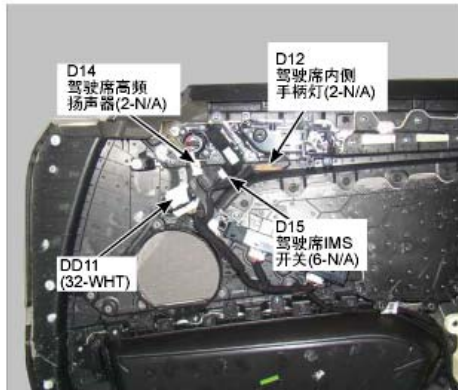
194.驾驶席车门装饰板
